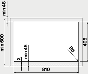
Dimensioni foro
