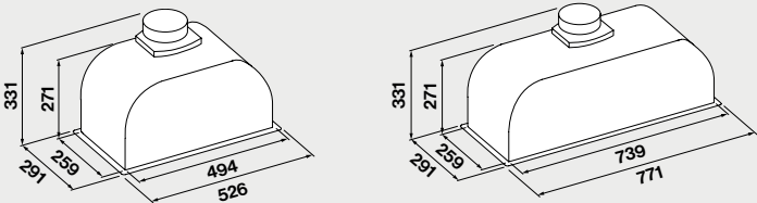
Foro per incasso 50 cm: 262 x 506 mm 70 cm: 262 x 751 mm
