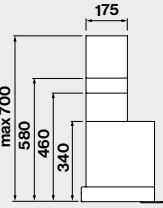
Vista laterale con camino opzionale
