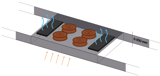
Filtrazione Multi-Air. 4 motori ultracompatte e 2 filtri Carbon.Zeo
