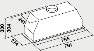
Foro per incasso 245 x 762 mm
