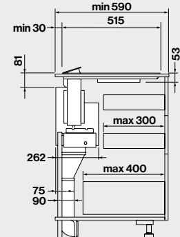
Vista laterale con motore in posizione anteriore
