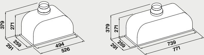
Foro per incasso 50 cm: 506 mm x 262 mm 70 cm: 751 mm x 262 mm
