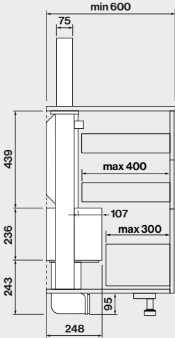
Dimensioni foro
