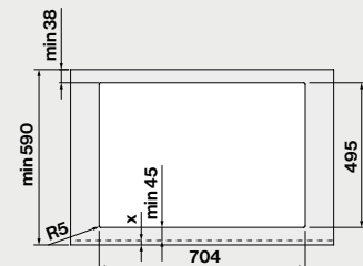
Dimensioni foro
