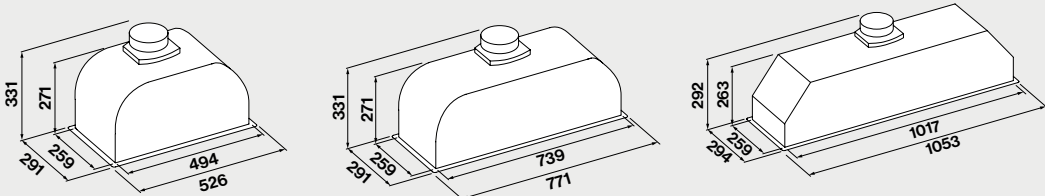
Foro per incasso 50 cm: 262 x 506 mm 70 cm: 262 x 751 mm 105 cm: 262 x 1029 mm
